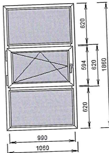
Изделие №2 Количество 1 шт. XS 358.01 Atex рама ПВХ XS 358.03 Atex имп. АТЕХ XS 358.02 Atex ств. Atex 58 мм *СПО 24мм AL Top-N Окно
