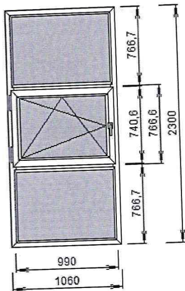
Изделие №1 Количество 8 шт. XS 358.01 Atex рама ПВХ XS 358.03 Atex имп. АТЕХ XS 358.02 Atex ств. Atex 58 мм *СПО 24мм AL Top-N Окно
