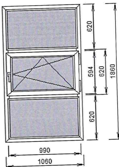
Изделие №3 Количество 1 шт. XS 358.01 Atex рама ПВХ XS 358.03 Atex имп. АТЕХ XS 358.02 Atex ств. Atex 58 мм *СПО 24мм AL Top-N Окно
